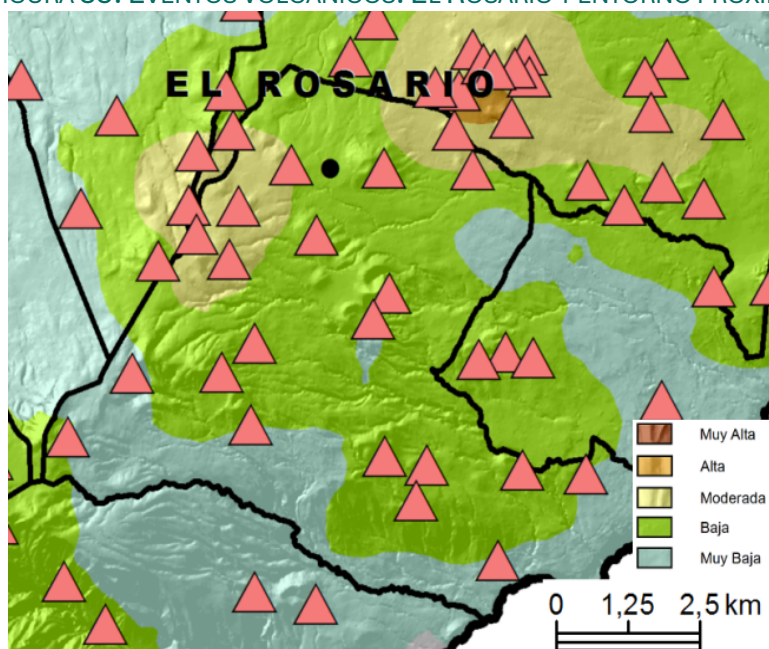
FIGURA 35. EVENTOS VOLCÁNICOS. EL ROSARIO Y ENTORNO PRÓXIMO
