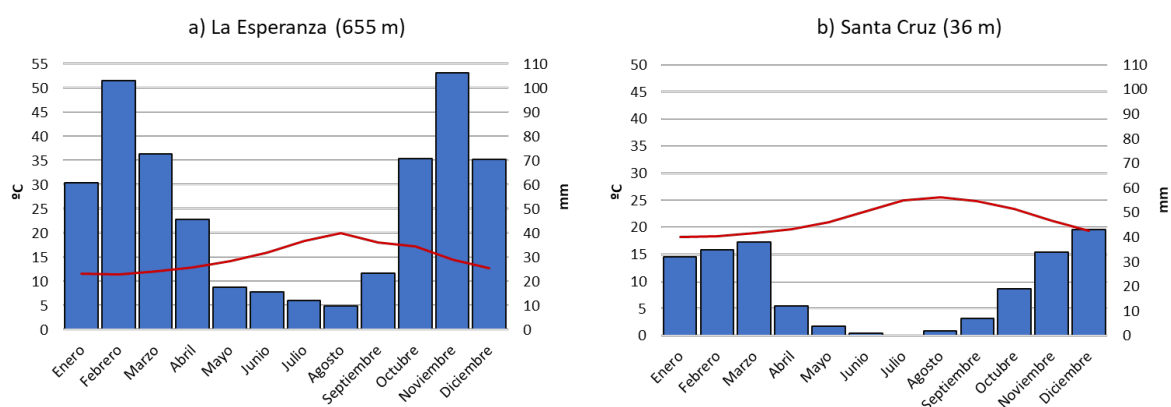
FIGURA 5. CLIMOGRAMAS. A) LA ESPERANZA- SECTOR MEDIANÍAS ; B) SANTA CRUZ DE TENERIFE - SECTOR DE COSTA
