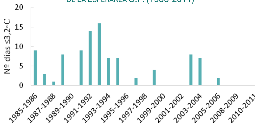
FIGURA 34. NÚMERO DE DÍAS QUE NO SUPERARON LOS 3,2°C EN LA ESTACIÓN METEOROLÓGICA DE LA ESPERANZA C.F. (1986-2011)
