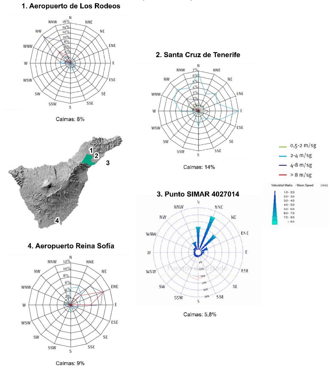
FIGURA 31. ROSAS DE VIENTOS DE 1) AEROPUERTO DE LOS RODEOS (1971-2000); 2) SANTA CRUZ DE TENERIFE (1971-2000); 3) PUNTO SIMAR 4027014 (1958-2016); Y 4) AEROPUERTO REINA SOFÍA (1971-2000)
