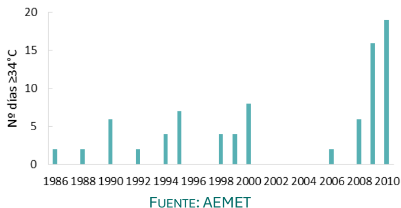
FIGURA 33A. NÚMERO DE DÍAS QUE SUPERARON LOS 34°C EN LA ESTACIÓN METEOROLÓGICA DE LA ESPERANZA C.F. (1986-2010) *NO EXISTEN DATOS DE LOS AÑOS 2001 Y 2007
