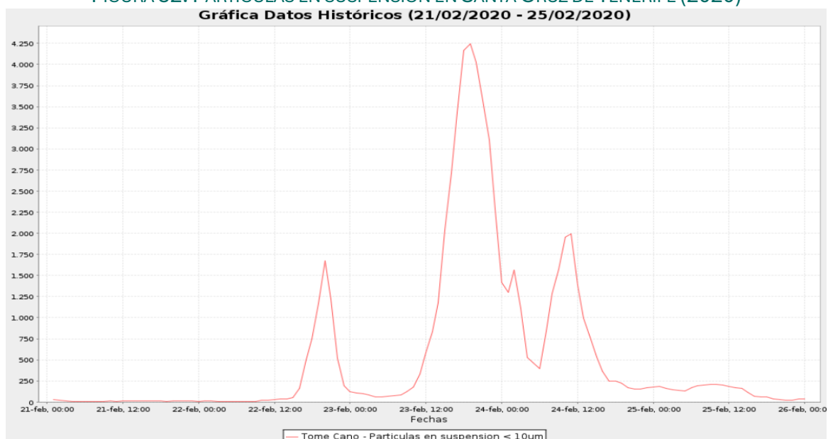
FIGURA 32. PARTÍCULAS EN SUSPENSIÓN EN SANTA CRUZ DE TENERIFE (2020)
