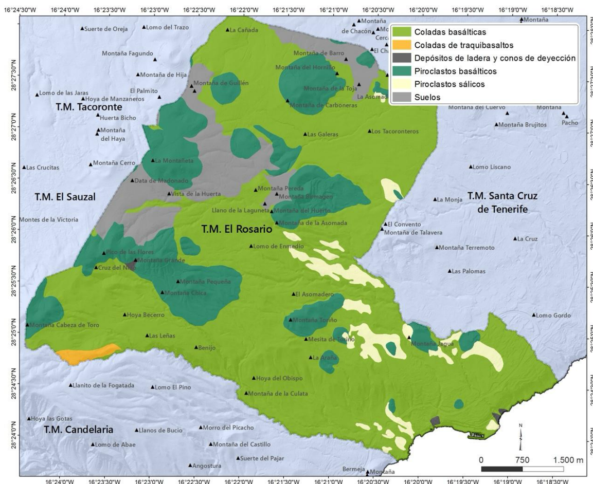
FIGURA 3. MAPA GEOLÓGICO DEL MUNICIPIO DE EL ROSARIO
