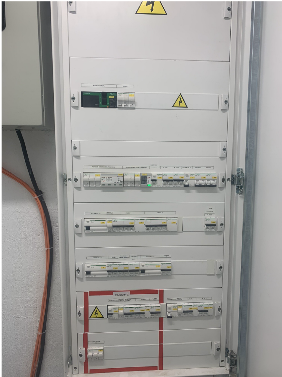
Cuadro eléctrico
