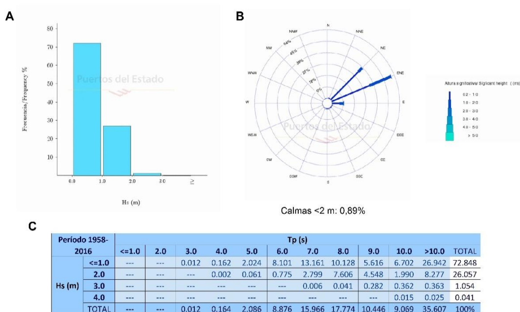
FIGURA 29. A) DISTRIBUCIÓN MEDIA ANUAL DE LA ALTURA DE OLA SIGNIFICANTE, B) ROSA DE OLEAJE Y C) TABLA DE ALTURA DE LA OLA SIGNIFICANTE Y PERÍODO PICO DE LA OLA, PARA EL PERÍODO 1958-2016 A PARTIR DEL PUNTO SIMAR 4027014
