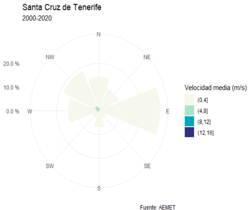
FIGURA 8. VELOCIDAD MEDIA Y DIRECCIÓN DE LOS VIENTOS EN SANTA CRUZ DE TENERIFE
