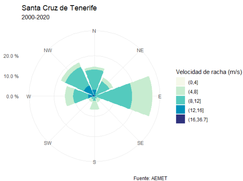
FIGURA 9. VELOCIDAD DE RACHA Y DIRECCIÓN DE LAS RACHAS MÁXIMAS DE VIENTO EN SANTA CRUZ DE TENERIFE
